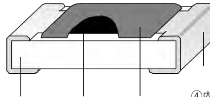
①基板 ②抵抗皮膜 ③保護膜 ④内部電極 中間電極 外部電極
