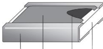
④内部電極 ③保護膜 ②抵抗皮膜 ①基板 中間電極 外部電極
