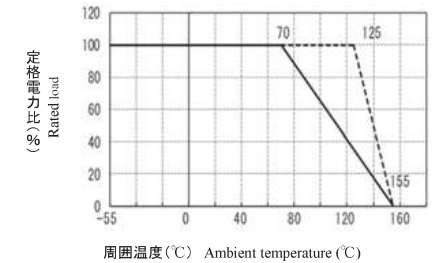
負荷軽減曲線 Load-Derating Curve
