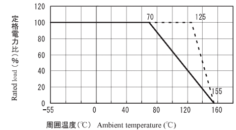
負荷軽減曲線 Load-Derating Curve
